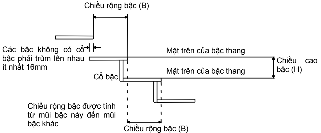
Hình 3.1. Đo chiều cao và chiều rộng bậc thang
